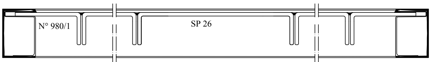
vaakaleikkaus 2-2
